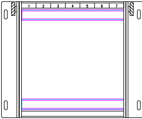
MPS-FMR-7MU-SD OD = 8.325" ID = 6.125" (7 MODULE UNITS)
