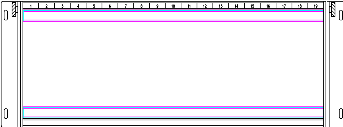
MPS-FMR-19MU-SD OD = 18.825" ID = 16.625" (19 MODULE UNITS)
