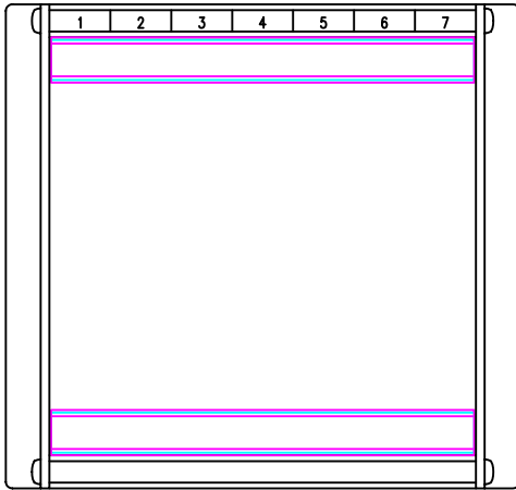
MPS-FMR-7MU OD = 7.125" ID = 6.125" <7 MODULE UNITS>
