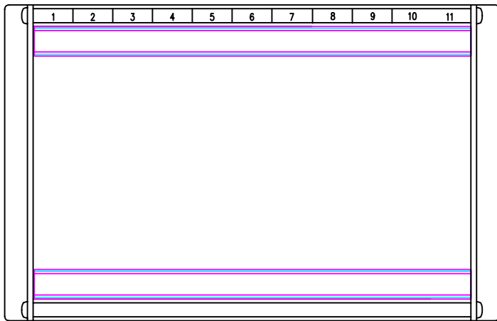
MPS-FMR-11MU OD = 10.625" ID = 9.625" <11 MODULE UNITS>
