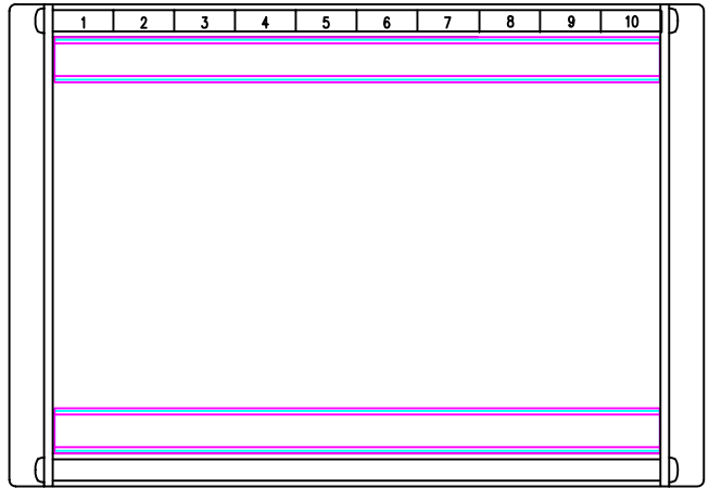
MPS-FMR-10MU OD = 9.75" ID = 8.75" <10 MODULE UNITS>
